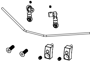
500205963 Stabi-Set vorne Anti roll bar front
